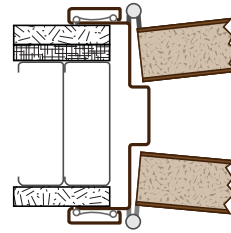
Jamb Hinge/Hinge
