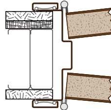
1B Jamb Hinge/Hinge
