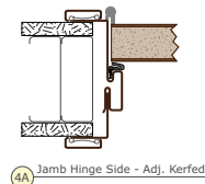
Jamb Hinge Side - Adj. Kerfed
