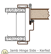
Jamb Hinge Side - Kerfed
