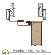
Header - Adj. Kerfed
