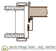
Jamb Hinge Side - Adj. Kerfed
