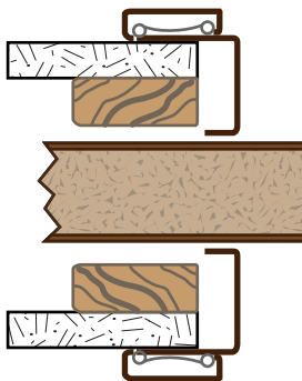
6A Jamb - Pocket Door Trim
