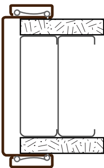
6U Jamb - No Stop
