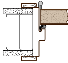
3A Jamb Hinge Side - Kerfed
